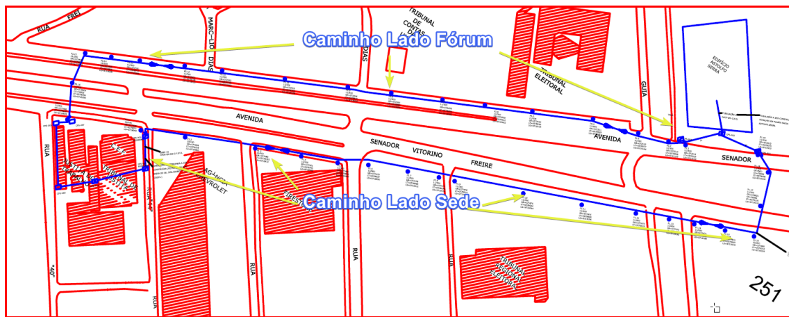
Figura 1 - Desenho do Anel Óptico do Tribunal
