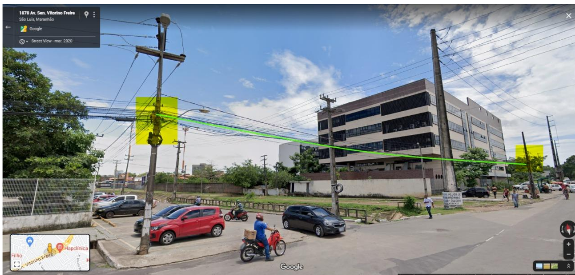
Figura 2 - Local de rompimento do cabo de fibra óptica
